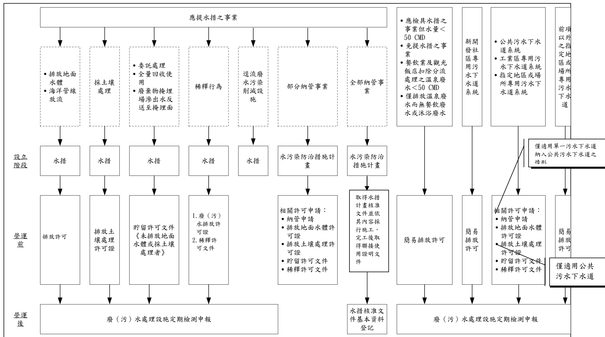
圖二 水污法各項許可申請時機
